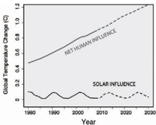
Figura 4. Influencia humana vs. Influencia solar desde 1980 y proyectado al 2030
